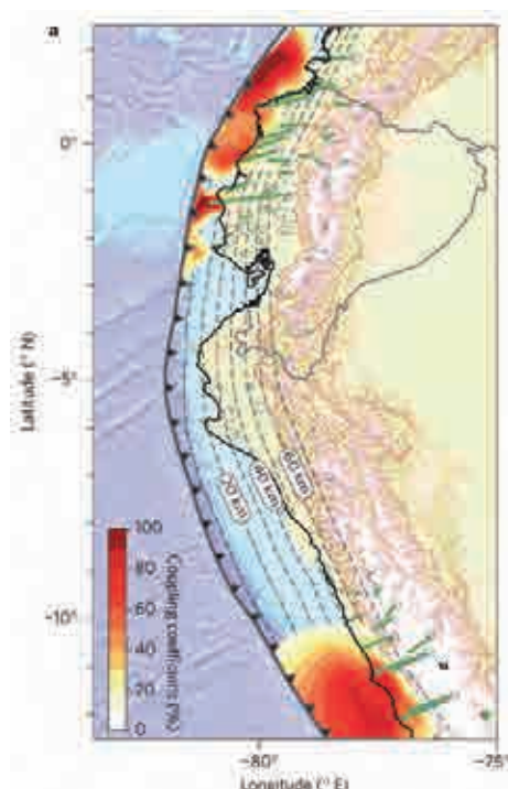
Fig. 5 : Modèle du couplage mécanique le long de l'interface de subduction, montrant le glissement asismique entre les zones de Lima et du Sud-Equateur ; vitesses GPS par rapport à l'Amérique du Sud © Géoazur. Nocquet et al. , 2014.
