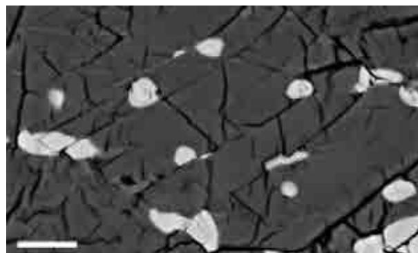
Fig. 2 : Expériences en laboratoire sur la rupture dynamique des roches et implications pour les processus précurseurs des tremblements de Terre (Schubnel et al. , 2013).
