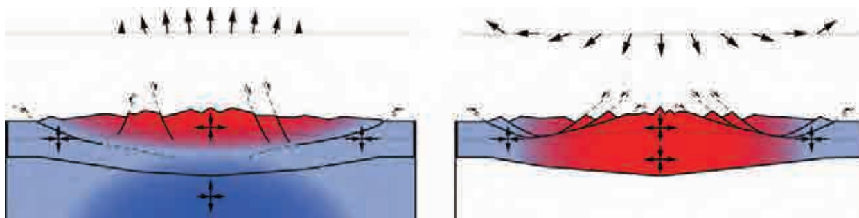
Fig. 4 : Extension induite par érosion des reliefs (à gauche), par effondrement gravitaire (à droite). La différence principale repose sur le champ de vitesse (composante horizontale plus rapide et subsidence au centre de la chaîne pour l'effondrement gravitaire). Il est à noter que dans le cas de l'extension induite par érosion, la croûte inférieure est en compression. Vernant et al. , 2013
