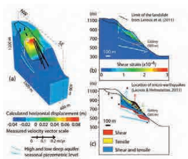
Figure 6 : Rôle des fluides dans la genèse d'un glissement de terrain (Cappa et al. , 2014).
