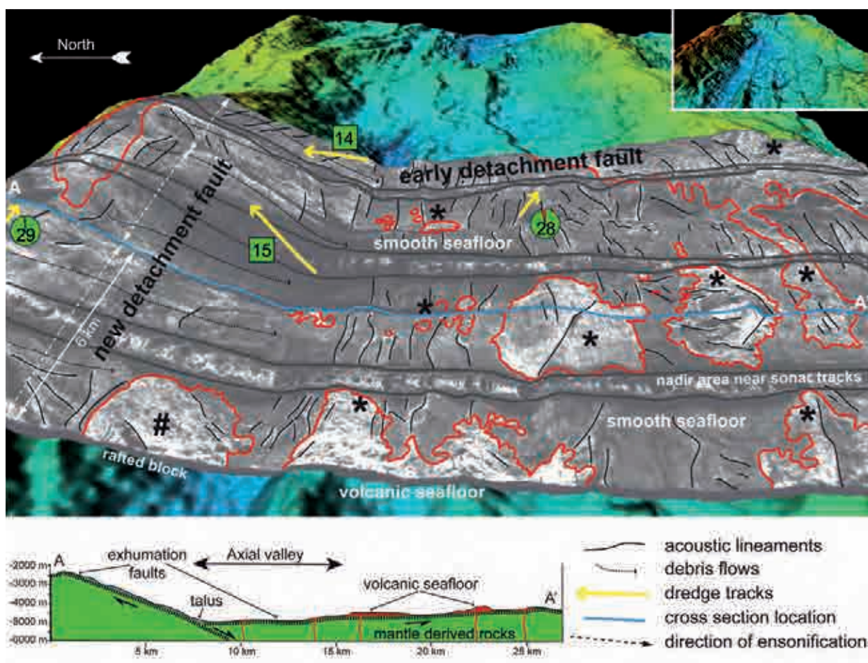
Fig. 1. La campagne océanographique SMOOTHSEAFLOOR (Marion Dufresne, dorsale sud-ouest indienne) a permis de mettre en évidence un nouveau mode de fonctionnement des dorsales océaniques, avec la mise à l'affleurement de roches du manteau sur des grandes surfaces et sur des longues périodes de temps. Ce processus d'exhumation du manteau, continu depuis au moins dix millions d'années, correspond donc à une accretion amagmatique, avec très peu de fusion et de production de basaltes. Sauter et al., Nature Geosciences , 2013.
