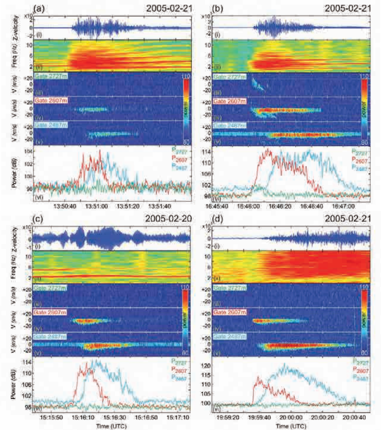
Fig. 3: Apports de l'analyse du bruit sismique à la prévision des éruptions volcaniques. Quatre événements sismiques représentatifs associés à un signal radar : a et b) explosion et séisme associé, c) trémor et d) émission sans signal sismique. (Valade et al., 2012).
