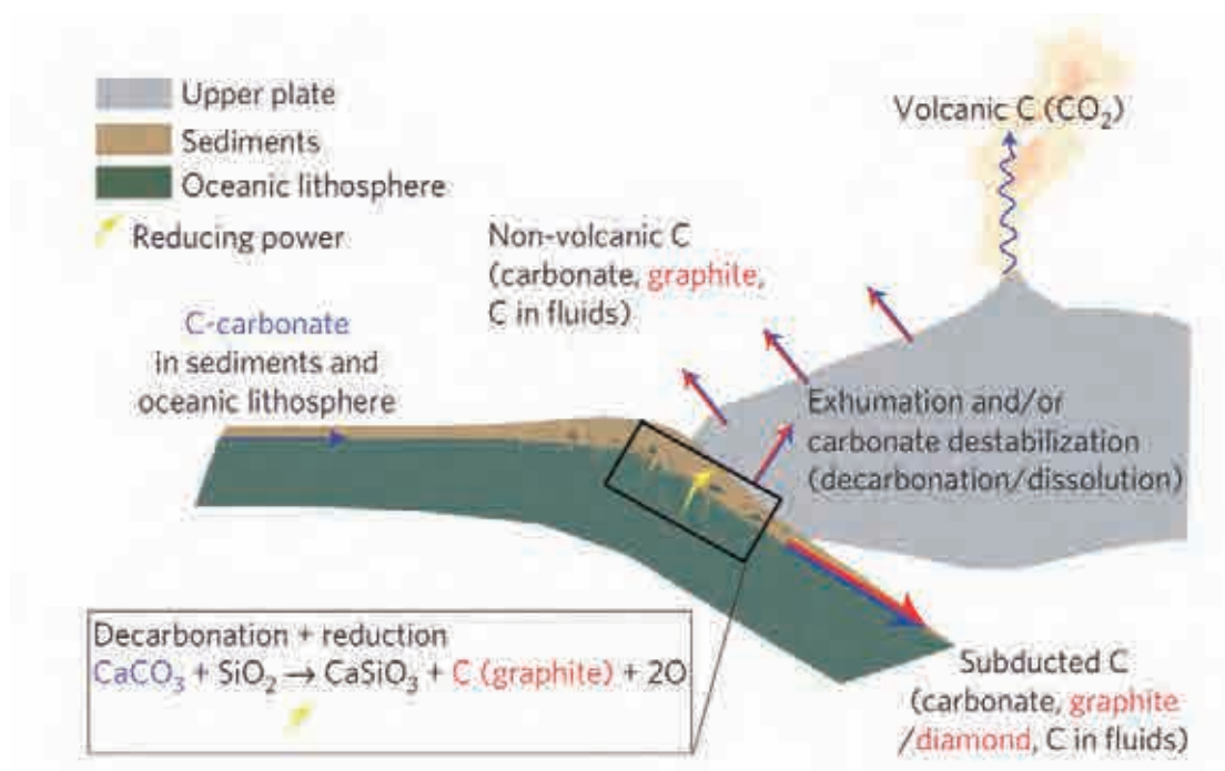
Fig. 4 – Devenir du carbone contenu dans les sédiments dans les zones de subduction. Environ 10% de la matière carbonatée des unités sédimentaires pourrait-être réduite en graphite et stockée pour être transportée en profondeur dans les zones de subduction (Galvez et al., 2013)
