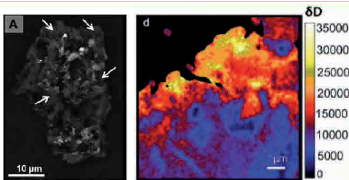
Fig. 3 : Image MEB et cartographie isotopique (D/H) par sonde ionique nanosims d'une micrométéorite ultra-carbonée (UCAMM) découverte dans les glaces antarctiques (Duprat et al. , 2010). Ces grains seraient d'origine cométaire.
