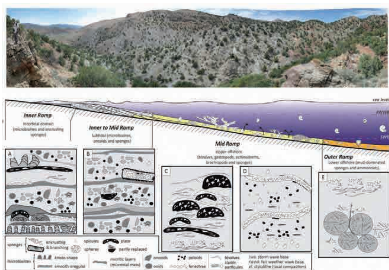
Fig. 2: Reconstitution des récifs à microbe et éponges riches en métazoaires Bayard et al. (2011) – Nature Geoscience 4, 693-697.
