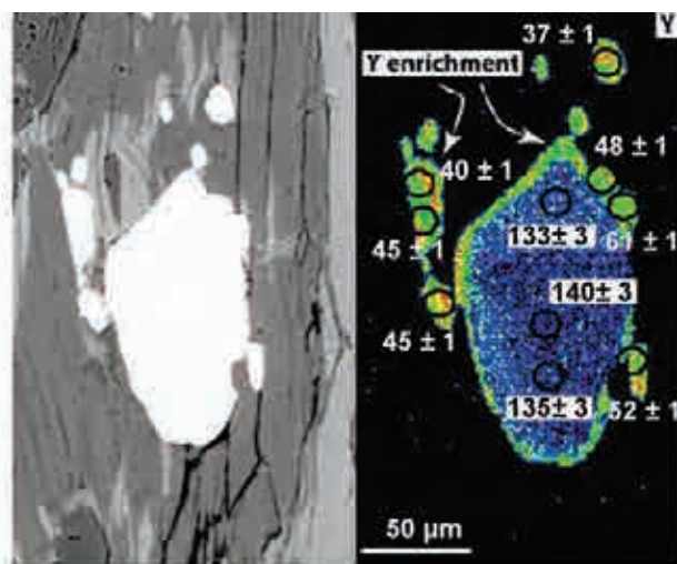
Fig. 1 : Textures, zonations en Y et âge U-Pb dans les monazites (Didier et al. , 2014).
