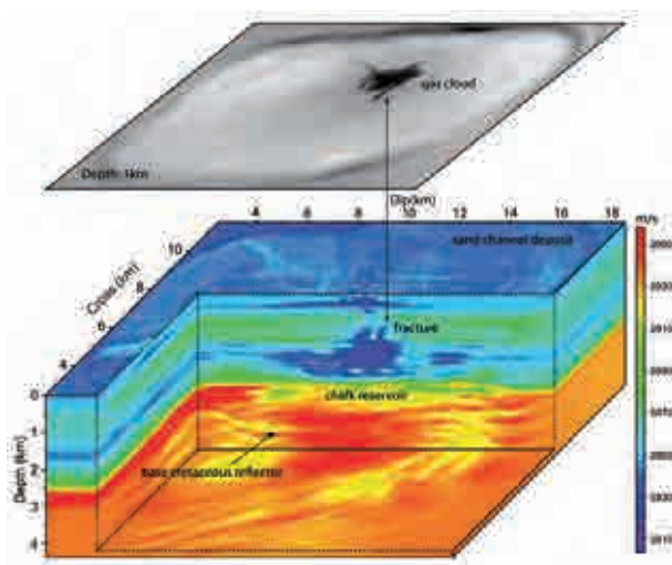
Fig. 1. L'inversion/tomographie multiparamétrique de grands volumes de données sismiques est une de tâches de l'imagerie sismique de haute résolution de l'échelle locale ou globale. Ici, interprétation des structures géologiques sous marines imagées : réservoir crayeux, fractures (injectées de gaz interdit par BP), nuage de gaz, dépôts sableux glaciaires, (poches et cheminée de gaz interdit par BP), scarifications laissées par des icebergs sur le paléofond (non illustré). Un réflecteur à faible vitesse à 500m de profondeur correspondant probablement à une zone d'accumulation de gaz. (Metivier et al., 2013)
