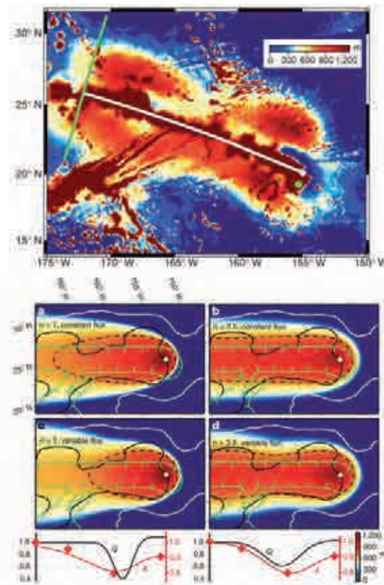
Fig. 4 : En haut, topographie résiduelle du bombement hawaïen; en bas, comparaison avec les résultats de différents modèles obtenus en changeant les caractéristiques non-linéaires de la rhéologie du manteau (Asaadi et al., Nature, 2011).
