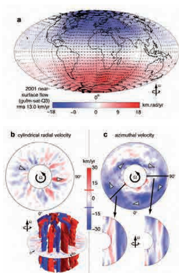
Fig. 6 : Un état possible de la dynamo terrestre pour l'époque 2001, rendant compte des observations magnétiques contemporaines (Aubert, G.Jl, 2013).
