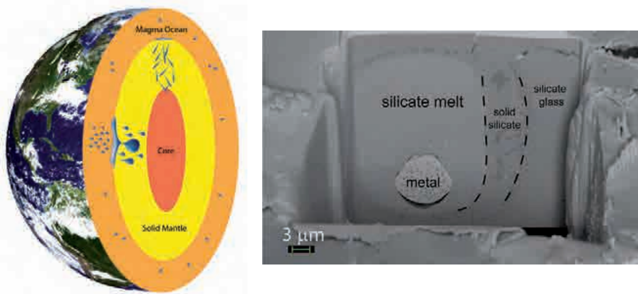
Fig. 1: Image en microscopie électronique d'un échantillon produit à haute pression (50 GPa) et haute température (3500 °C). Son analyse chimique permet de mieux connaître la répartition du chrome et du vanadium entre les liquides métalliques silicatés et au cours de la formation du noyau. La présence d'oxygène en quantité dans le métal permet d'expliquer les abondances de ces éléments dans le manteau terrestre et montre qu'on peut former un noyau riche en oxygène. (Siebert et al. , Science, 2013).
